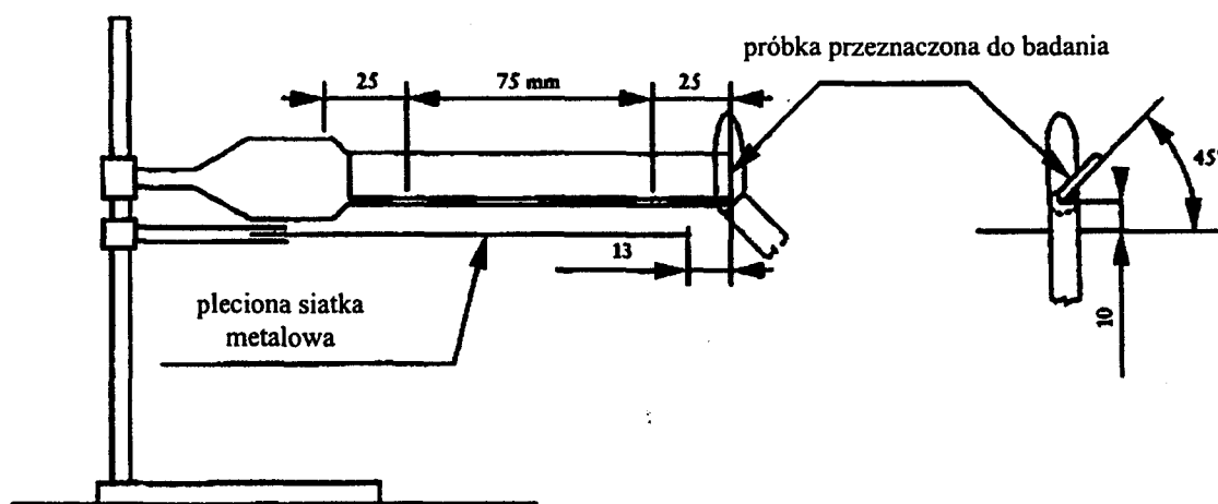
Aparatura badawcza
