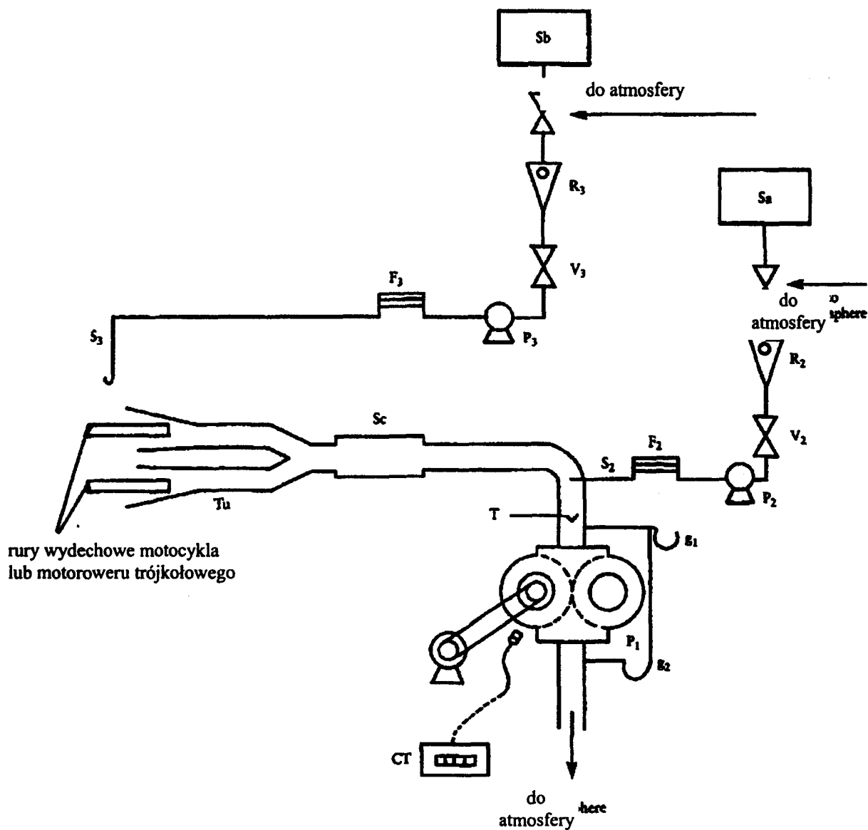
Przykład nr 1 systemu odbioru spalin
